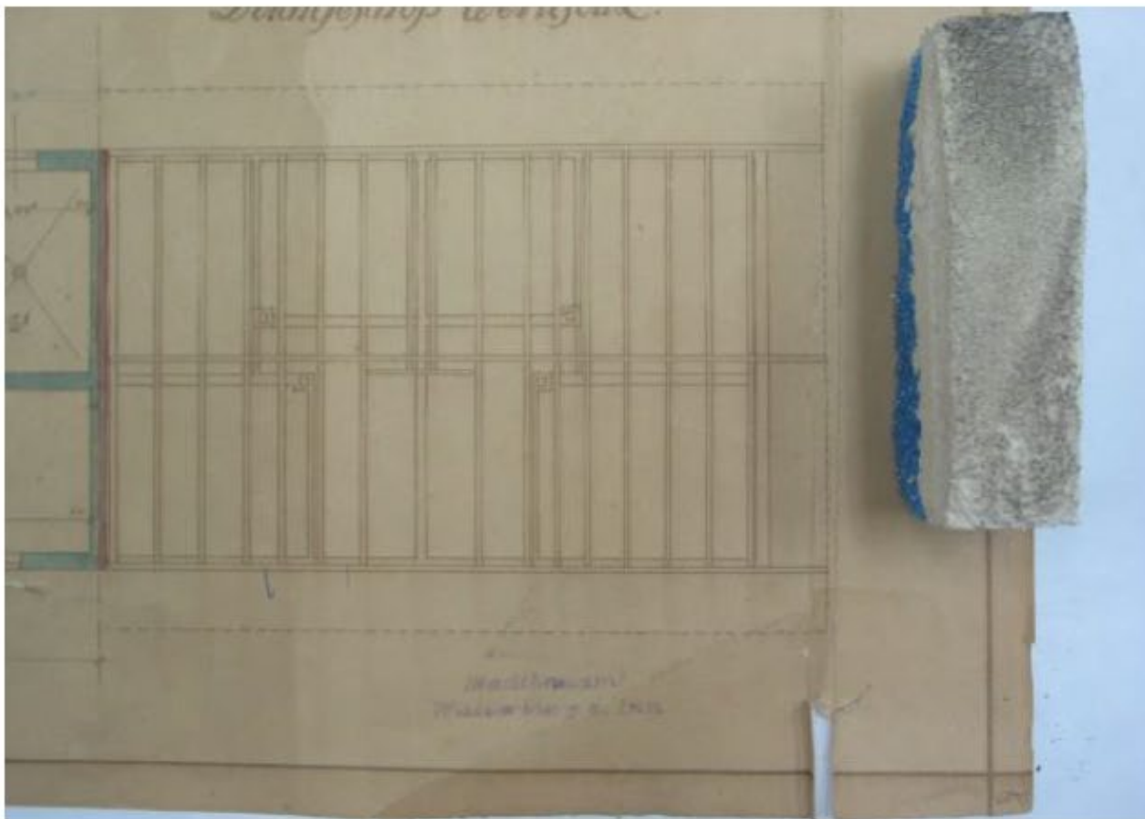
Beispiel der Oberflächenreinigung mit AKAPAD- Schwamm (links) Materialien zur Oberflächenreinigung (rechts)
