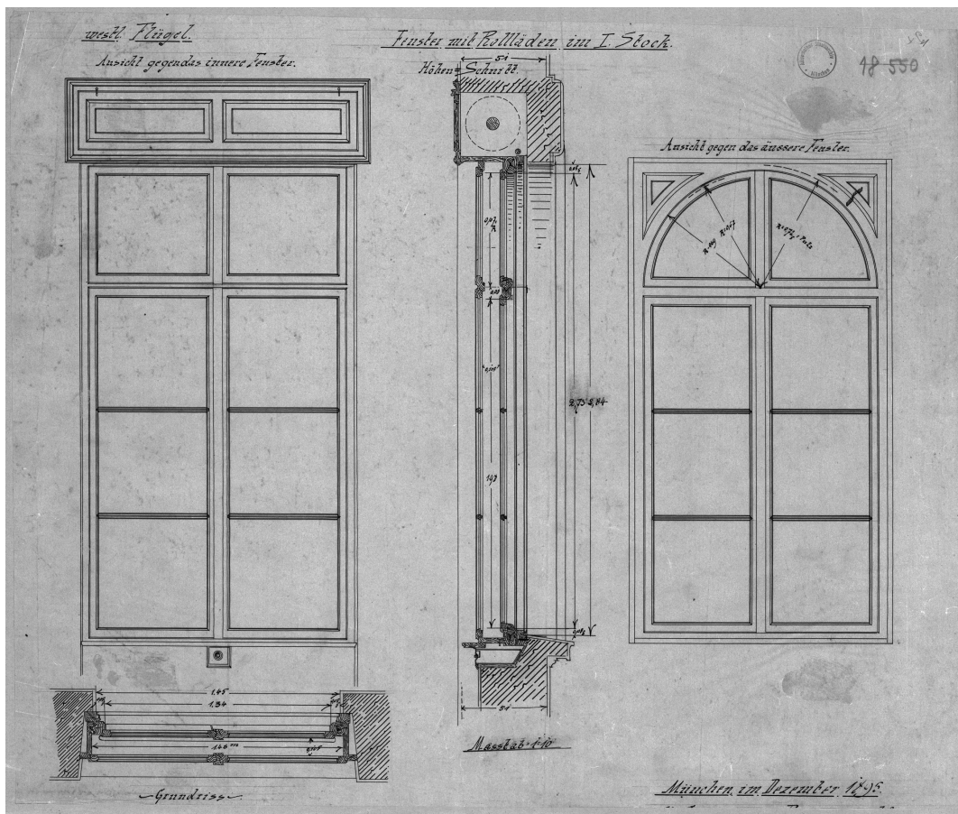
Entwurf von 1895 für Fenster an der Westfassade (mit Rolläden) (Bayerisches Hauptstaatsarchiv, OBB Karten und Pläne 3928).
