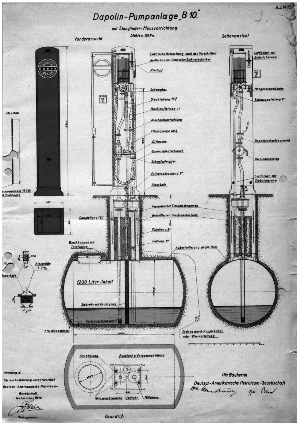
Technische Zeichnung einer Dapolin-Pumpanlage mit Einzylinder-Messvorrichtung (Staatsarchiv Coburg, Gewerbeaufsichtsamt Nr. 127).
